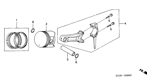
PISTON
