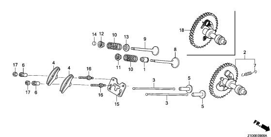
CAMSHAFT
